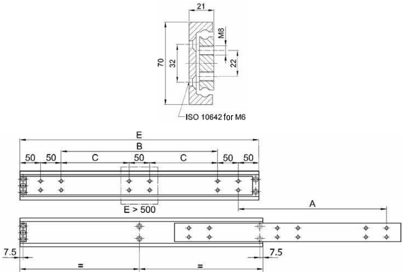
Load Table
