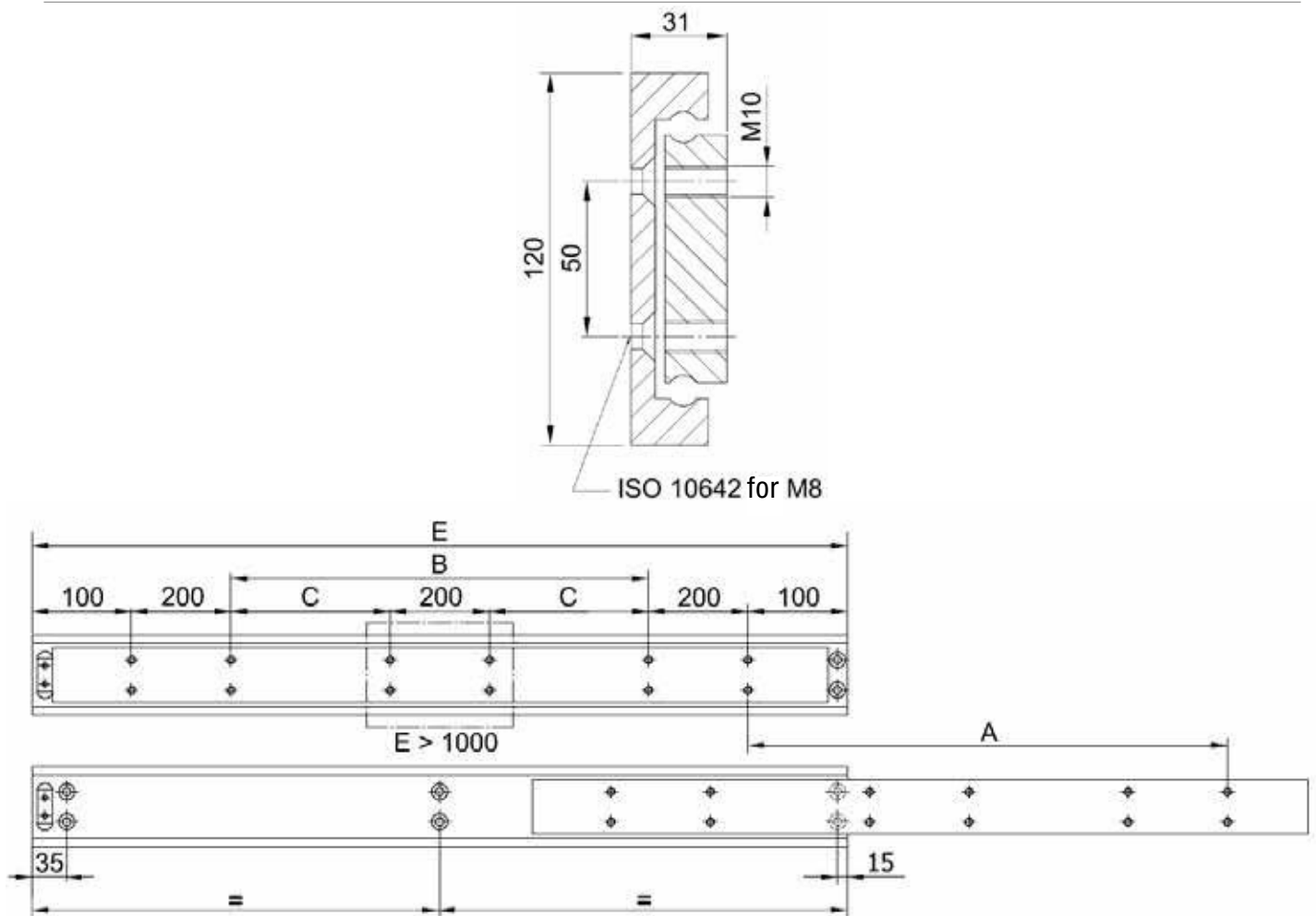
Load Table
